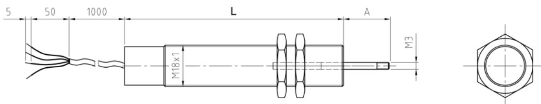
Anschluss: Kabel 1m Connection: Cable 1m
