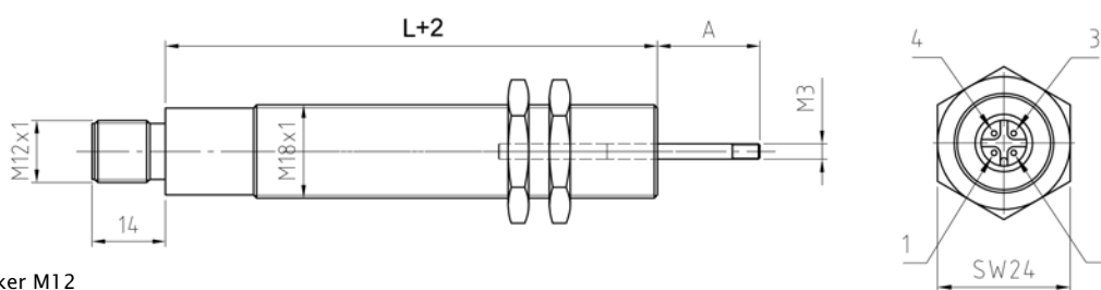
Anschluss: Stecker M12 Connection: Plug M12
